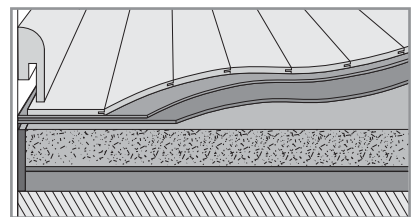
Паркет на материале Uno-Protect / ПВХ / минеральной стяжке
