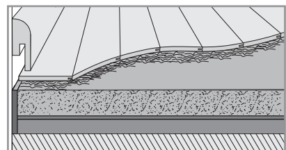
Полностью приклеенный паркет
