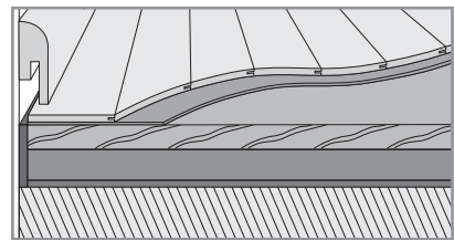
Паркет на материале Uno-Protect /
