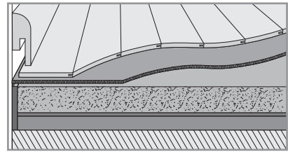
Паркет на материале Duo-Protect / минеральной стяжке
