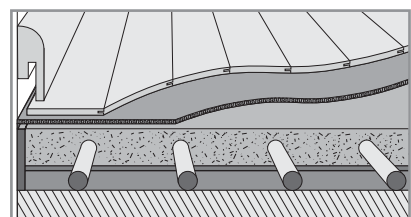
Паркет на материале Duo-Protect / на полах с подогревом горячей водой
